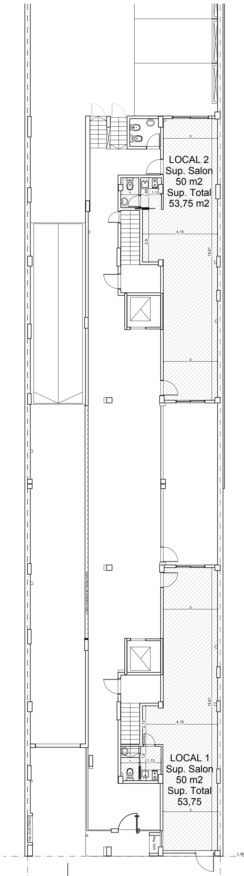
PLANTA BAJA ESC. 1-125
